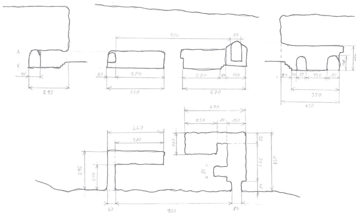
16. A C-bunker alaprajza és oldalnézetei
